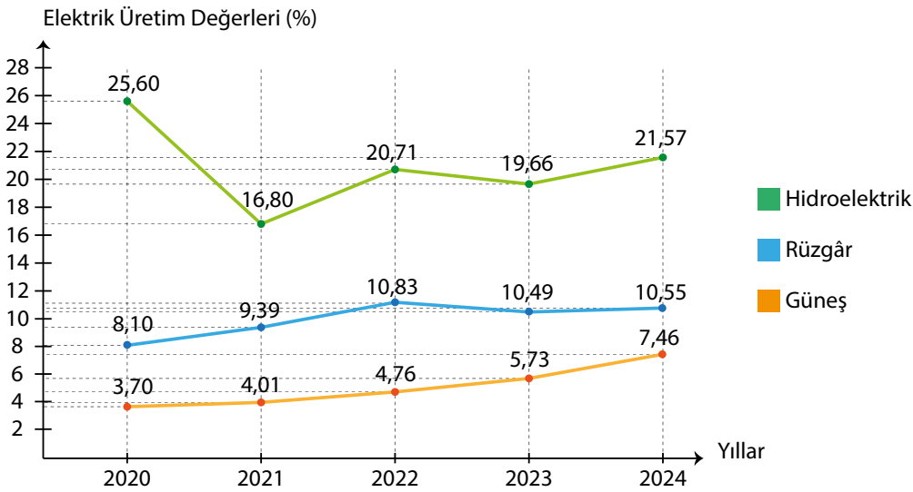
Grafik: Yenilenebilir Enerji Kaynaklarının Elektrik Üretim Değerleri
