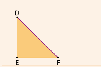
Şekil 2: İkizkenar Dik Üçgen
