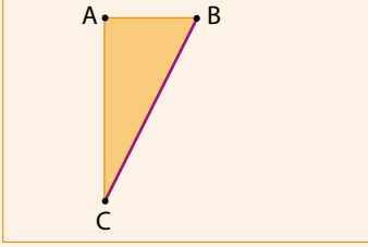
Şekil 1: Çeşitkenar Dik Üçgen
